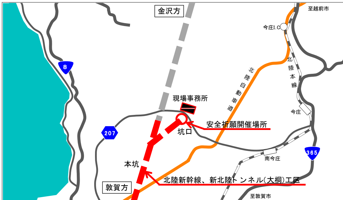
安全祈願会場詳細図
