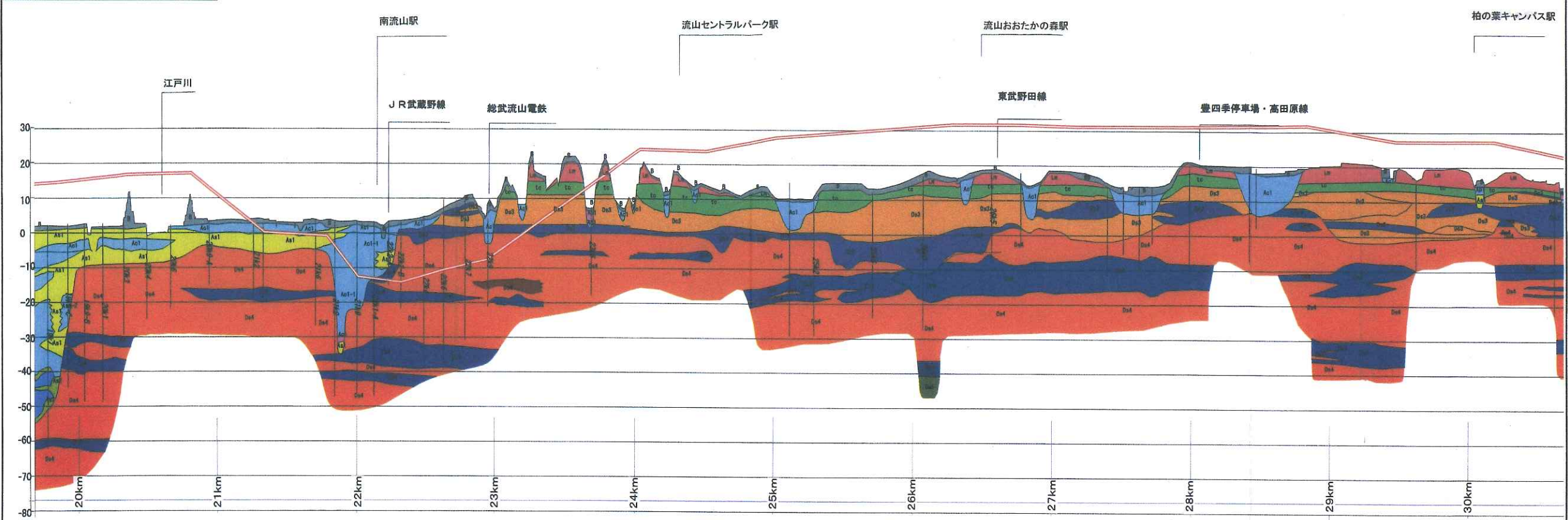
地質縦断面図 横 1:20,000 縦 1:800 20.0km~40km
