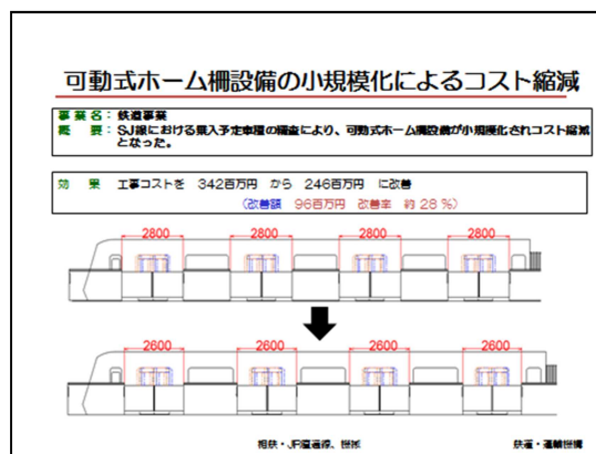
図 1.1.2-4 コスト削減の取組み例 （可動式ホーム柵設備の小規模化によるコスト削減）
