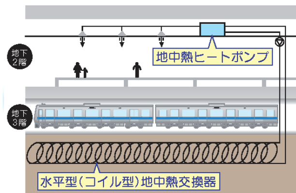
世田谷代田駅における 地中熱ヒートポンプシステム概念図
