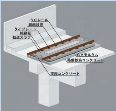
スラブ軌道概要図
