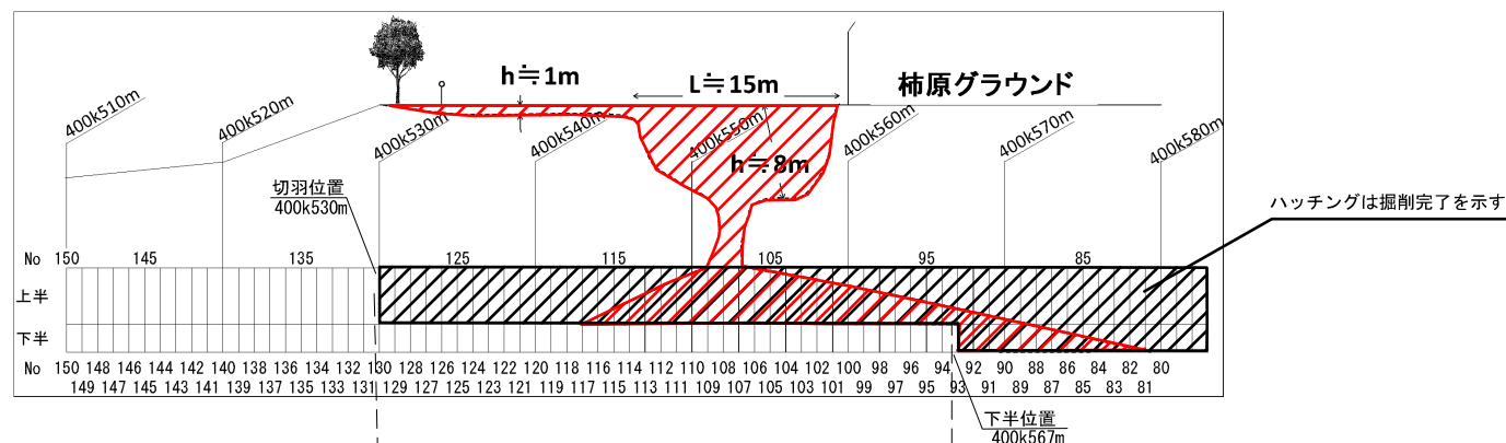
側面図
