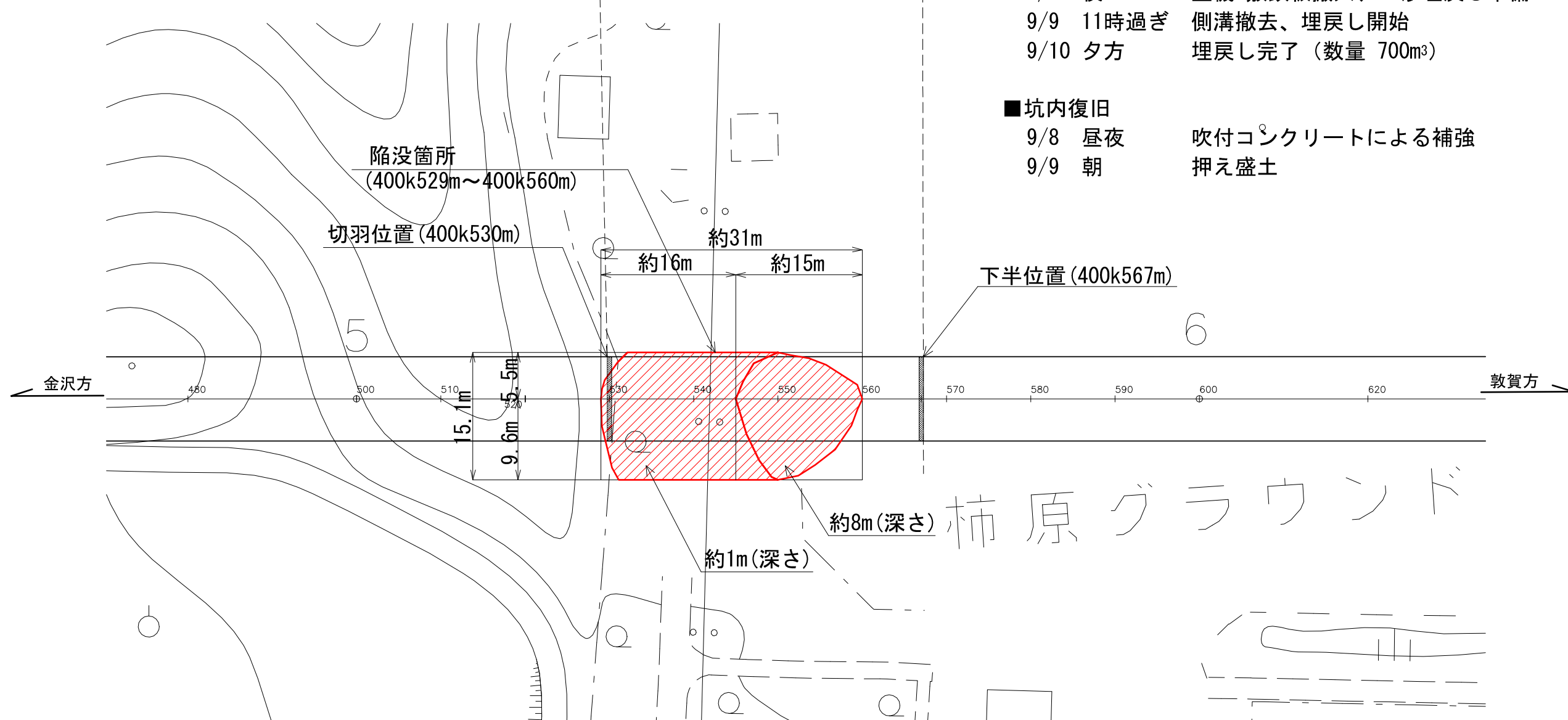
平面図
