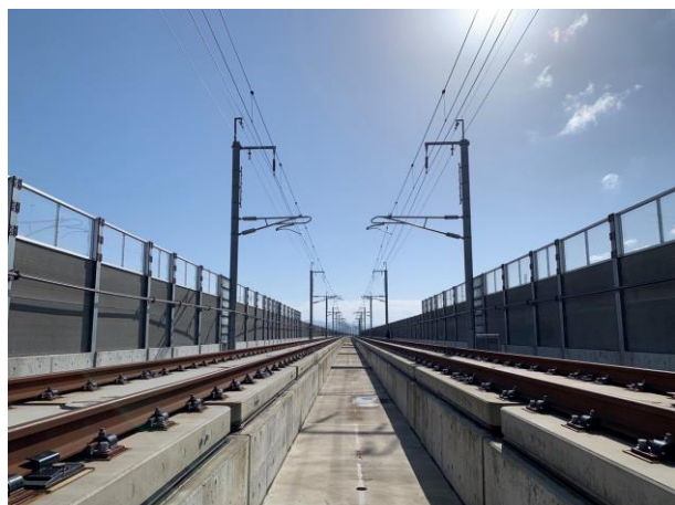
高架橋内観 (福井県)
