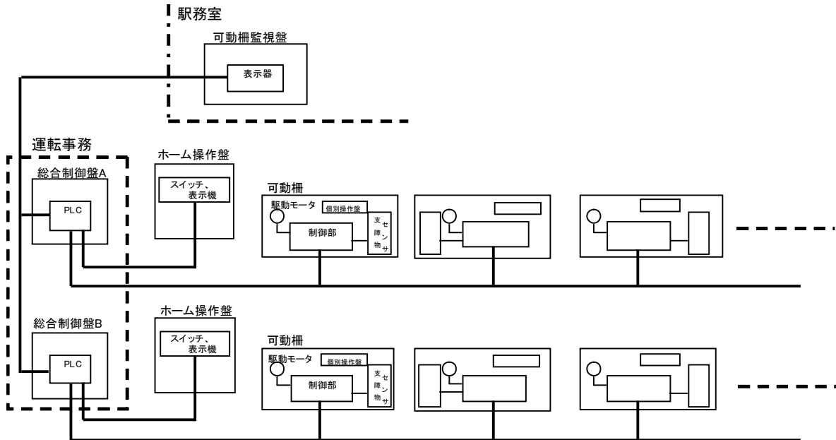
図 10.3.1 可動柵システム構成例
