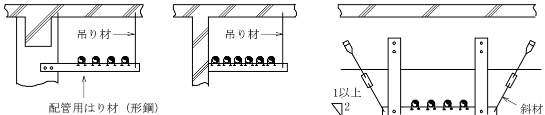
(4) 柱・壁等を利用する方法
