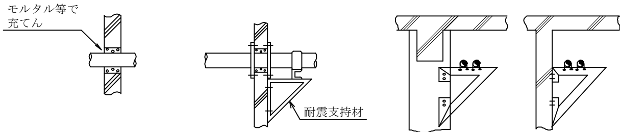
(1) はり・壁等の貫通部
