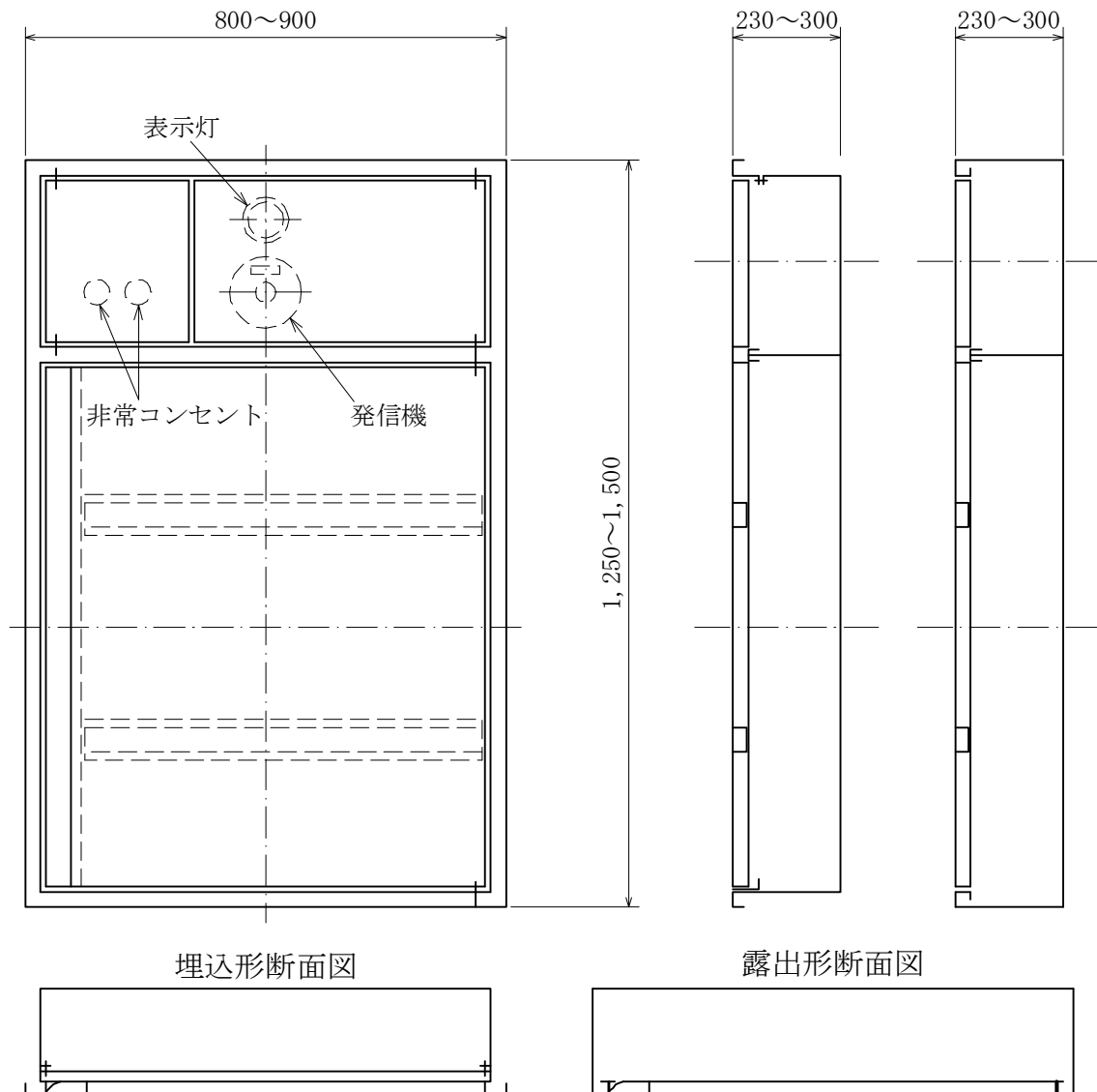
正面図
