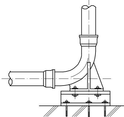
曲り部
