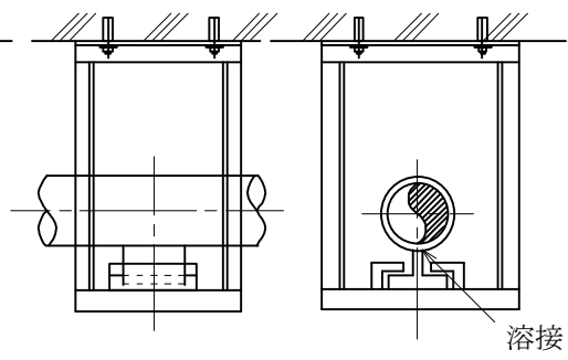
(2) ガイドシュー
