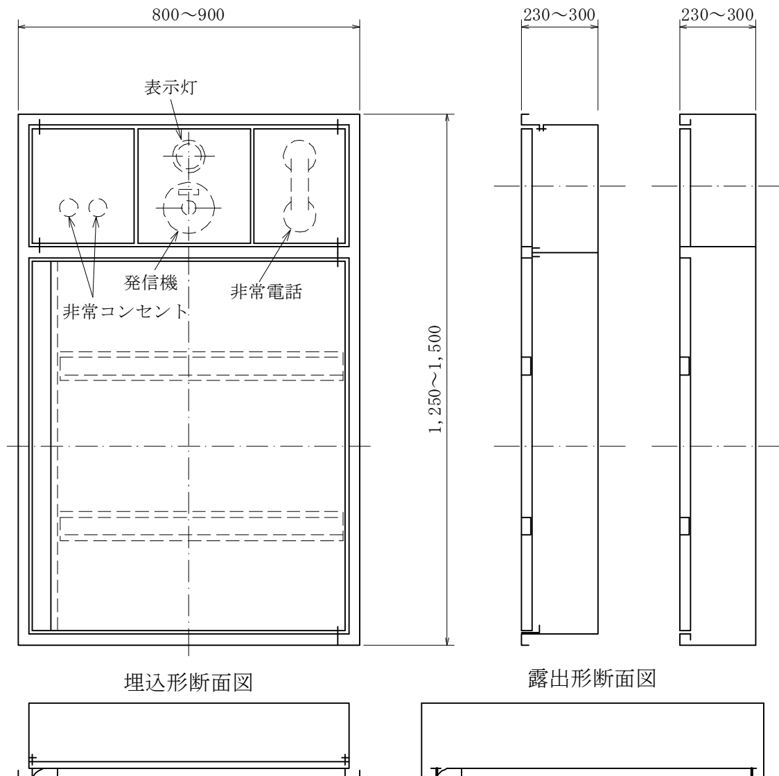
正面図
