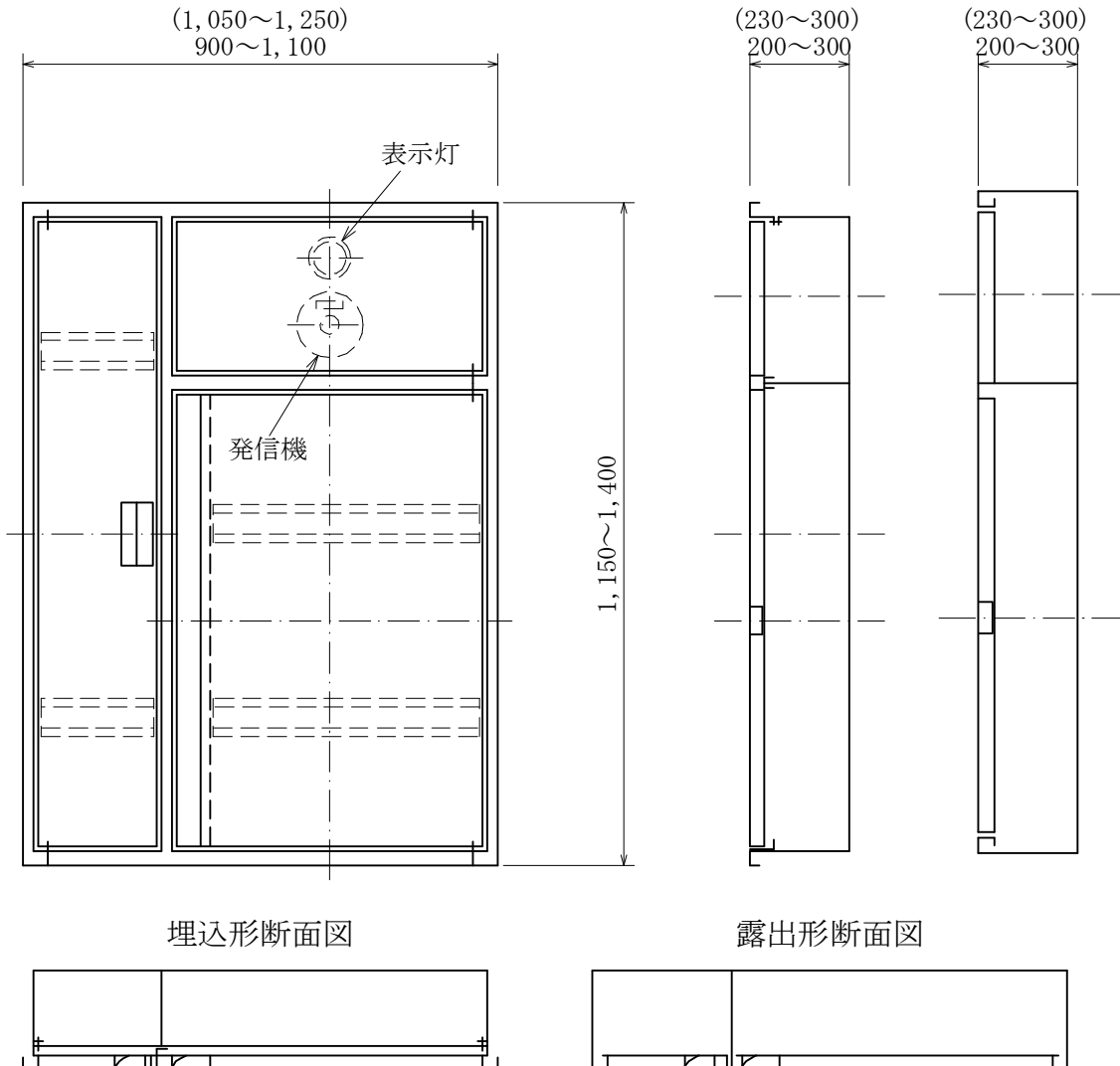
正面図
