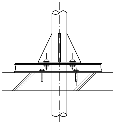
立面図
