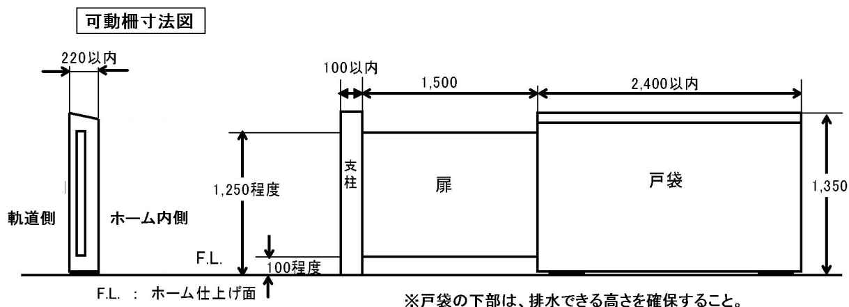
図 10. 2. 2 可動柵標準寸法図
