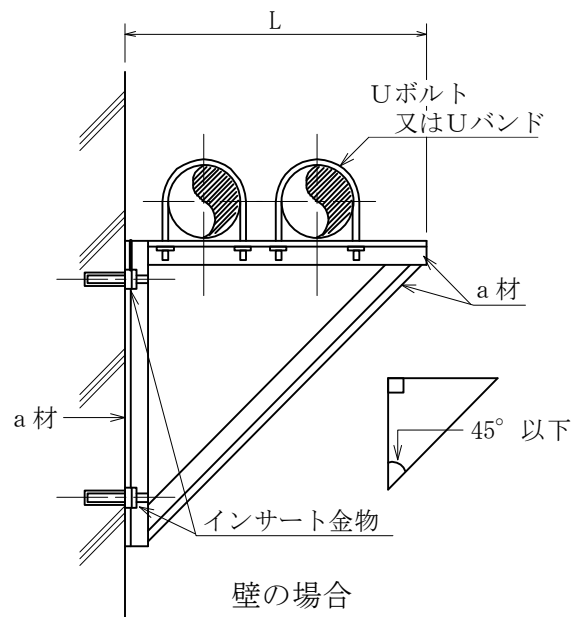
形鋼 複数管の場合
