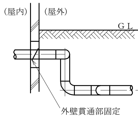
〔立面〕
