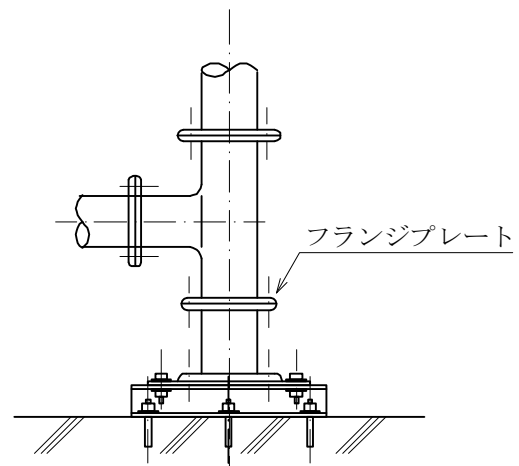
立面図
