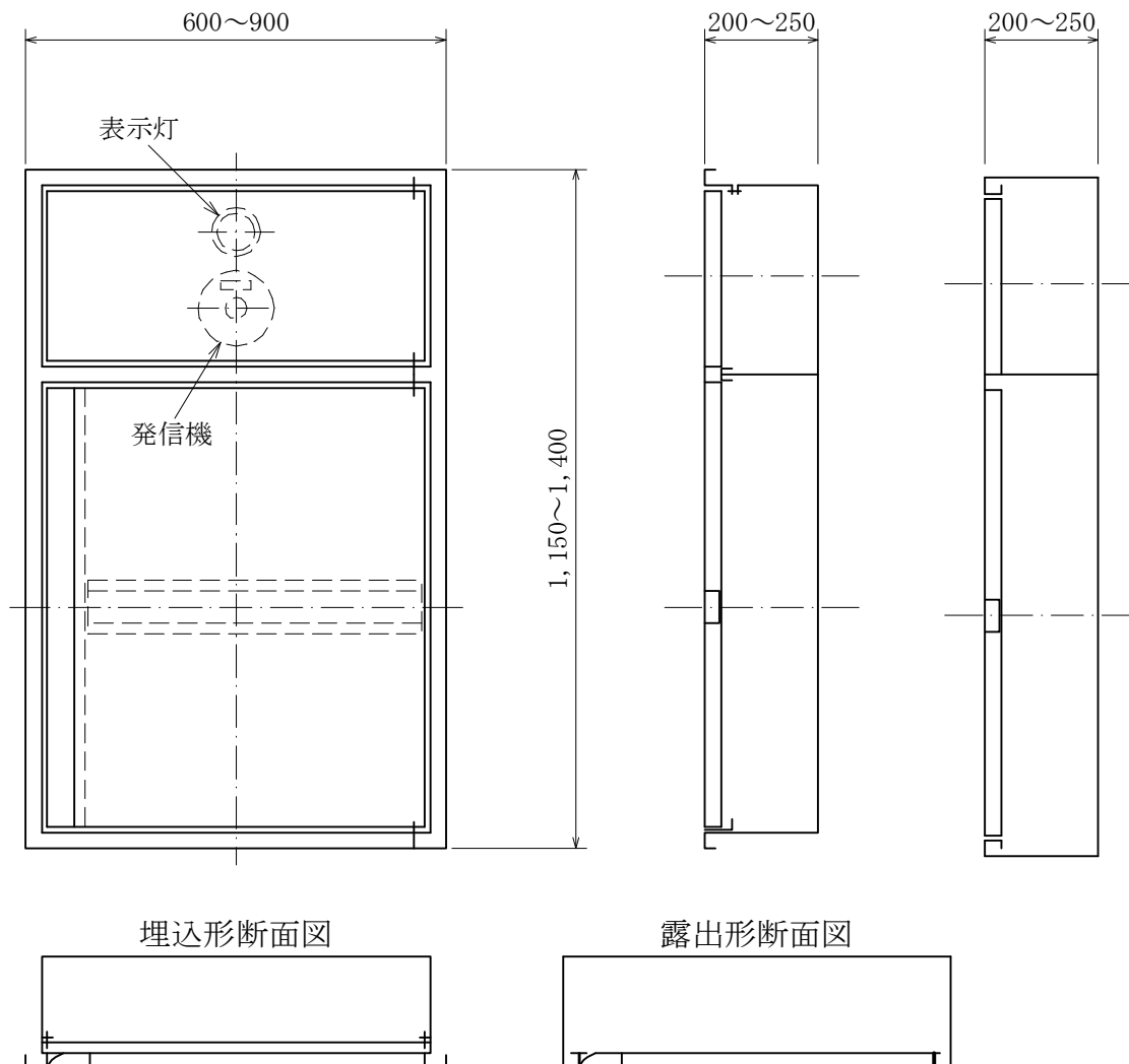
正面図
