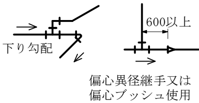
(f) リフト継手 (蒸気配管)
