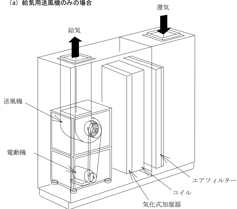
(a) 給気用送風機のみの場合
