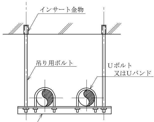
形鋼 複数管の場合
