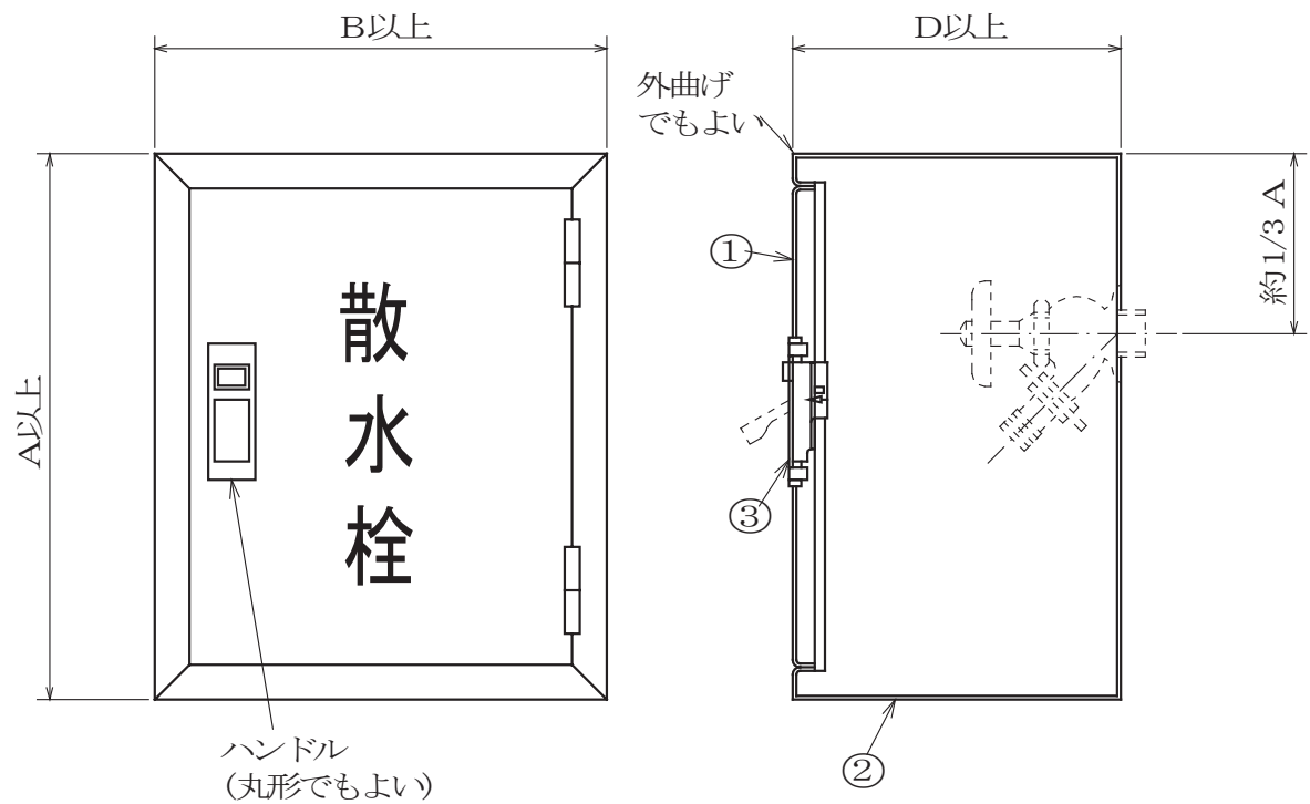
構成部品表
