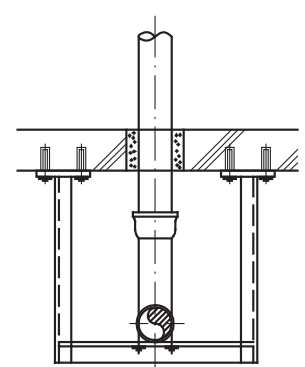
垂直部と曲り部
