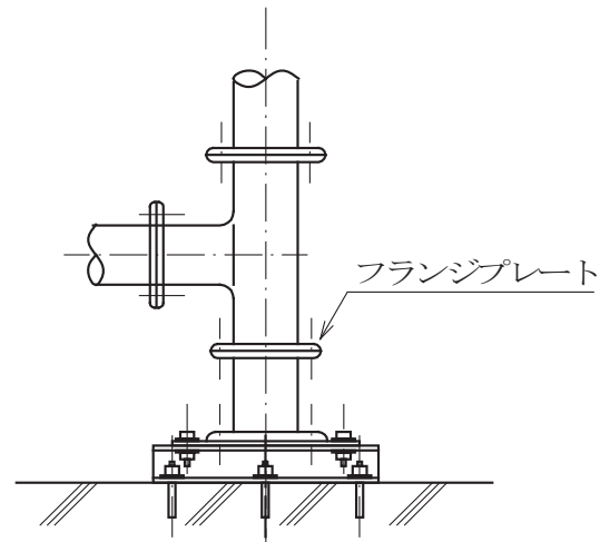
立面図
