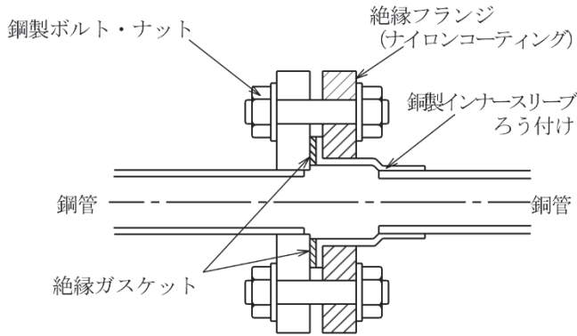
(1) 絶縁フランジの例
