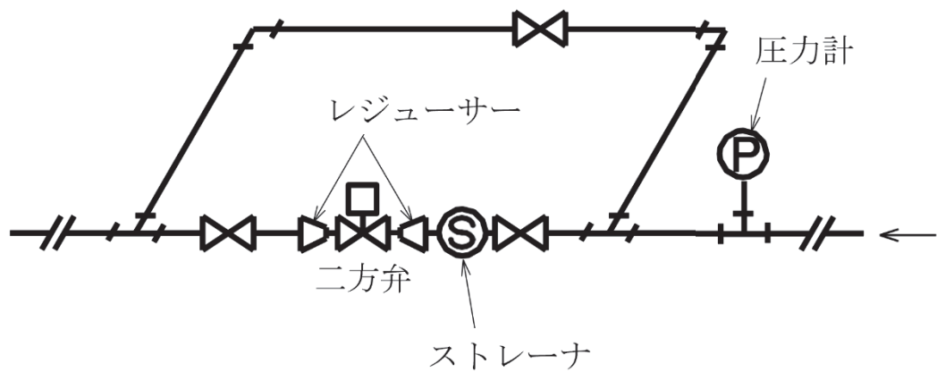
(b) 二方弁装置
