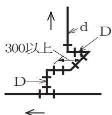
(a) 分岐(蒸気配管)
