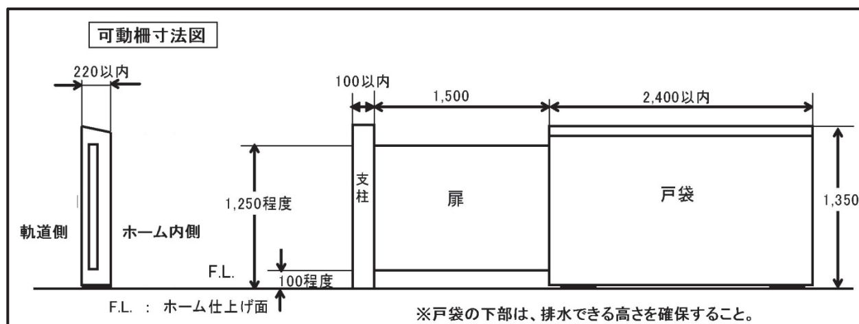
図 10.2.2 可動柵標準寸法図
