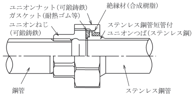
(イ) ステンレス鋼管と鋼管
