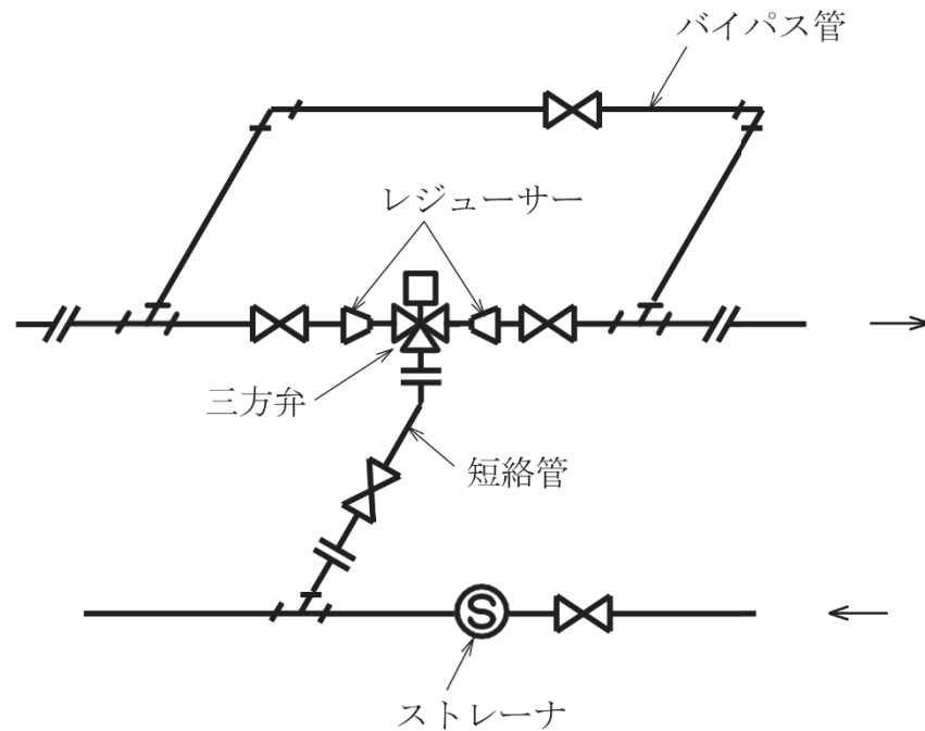
(a) 三方弁装置
