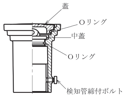
(d) 漏えい検査管口
