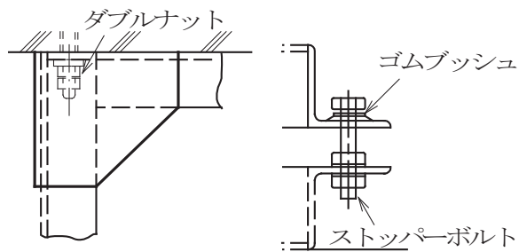
A部隔詳細図
