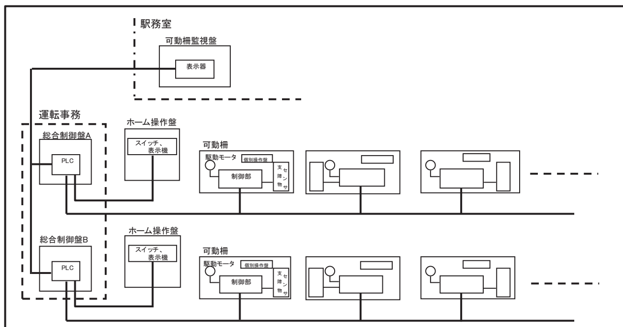
図 10.3.1 可動柵システム構成例
