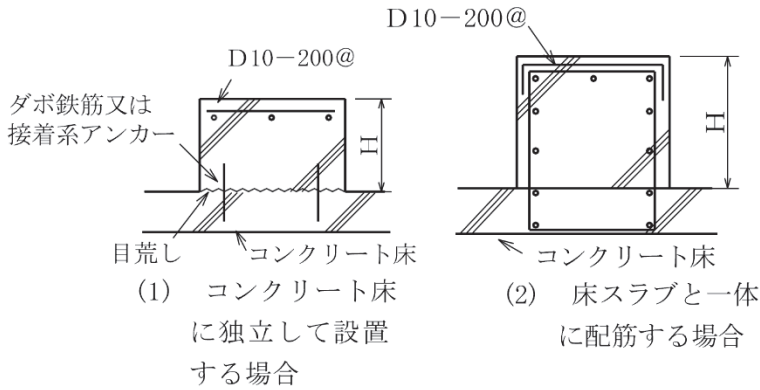
(a) 基礎の高さと配筋要領
