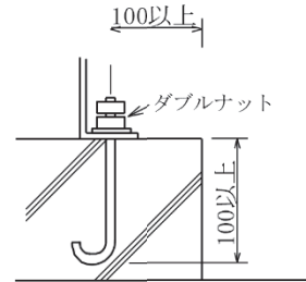
(b) アンカーボルトの取付位置等
