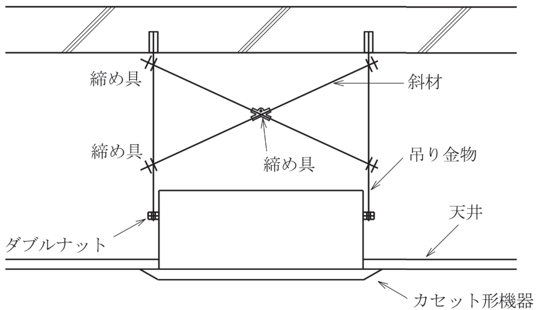
(b) カセット形機器の振れ止めの例
