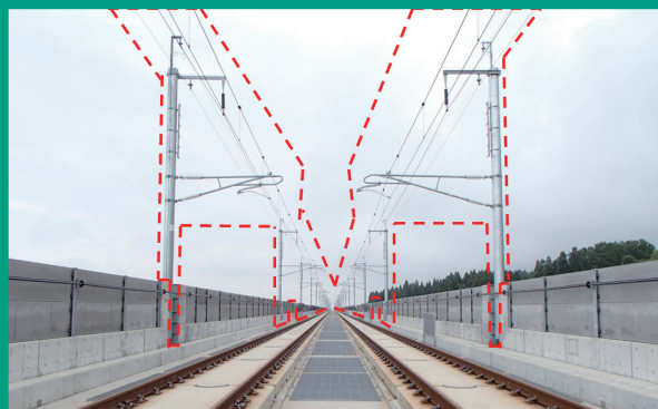
電車線工事の範囲(赤点線囲み部分)
