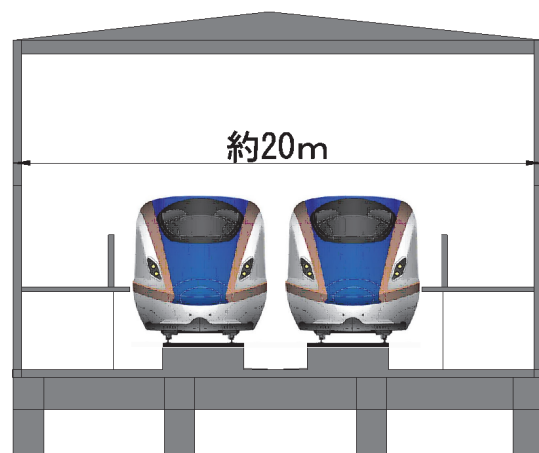
地上駅 ※2面2線の場合
