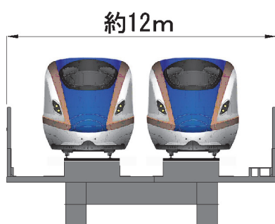
高架橋・橋梁
