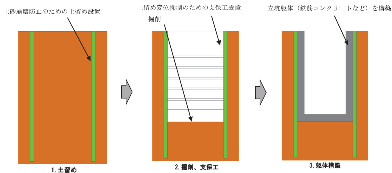
図 3-3-13 立坑の施工イメージ
