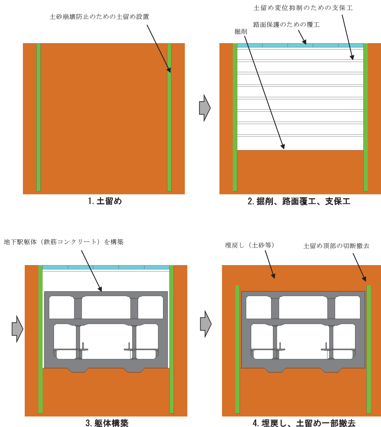
図 3-3-10 地下駅の施工イメージ ※2 面 2 線の地下駅、開削工法の場合
