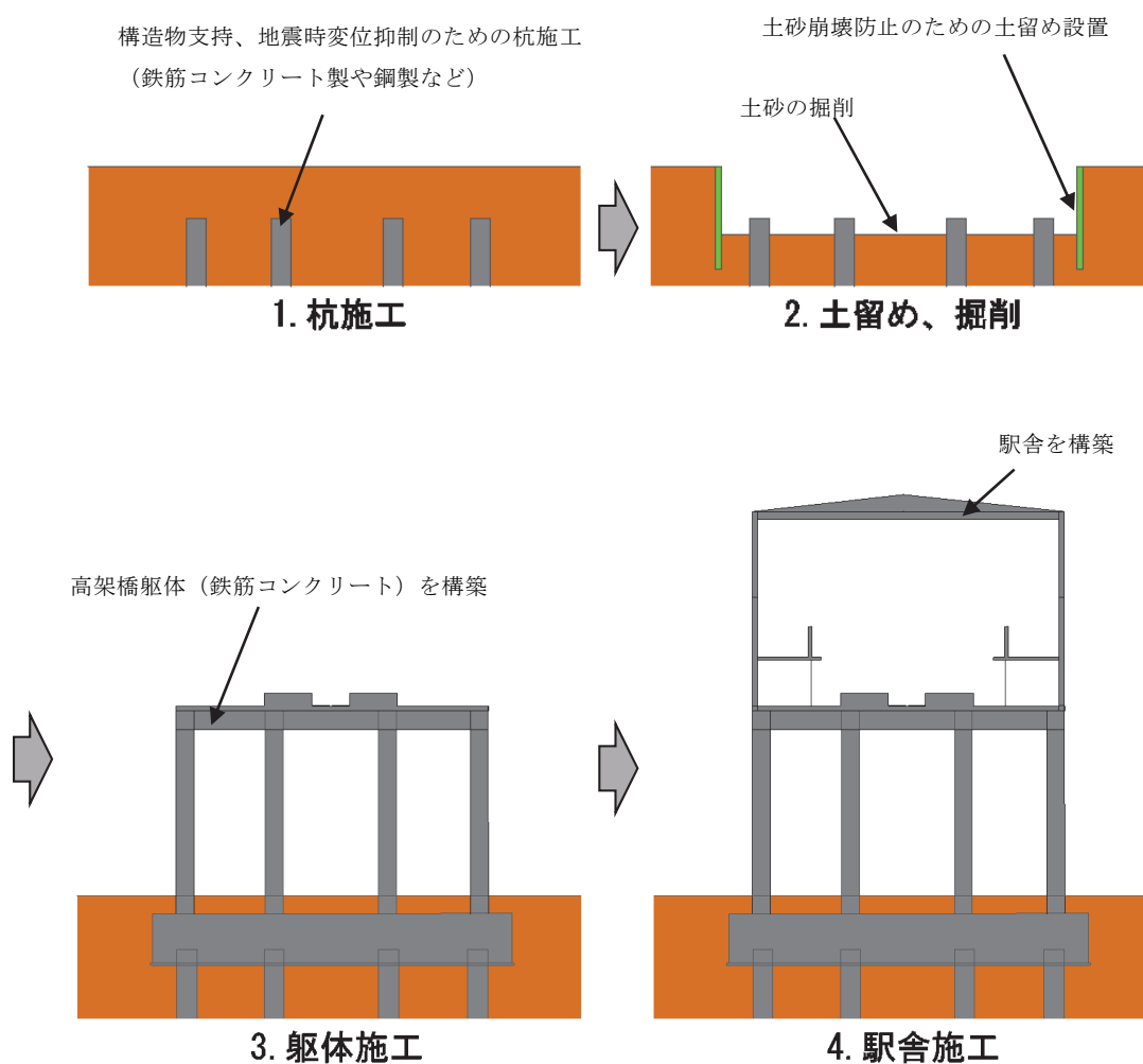
図 3-3-9 地上駅の施工イメージ ※2 面 2 線の地上駅、場所打ち工法の場合
