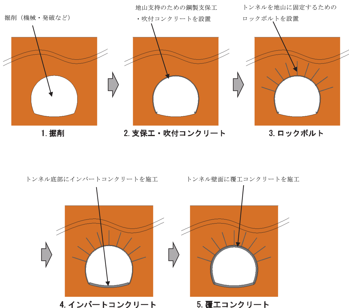
図 3-3-11 山岳トンネルの施工イメージ ※NATM 工法の場合
