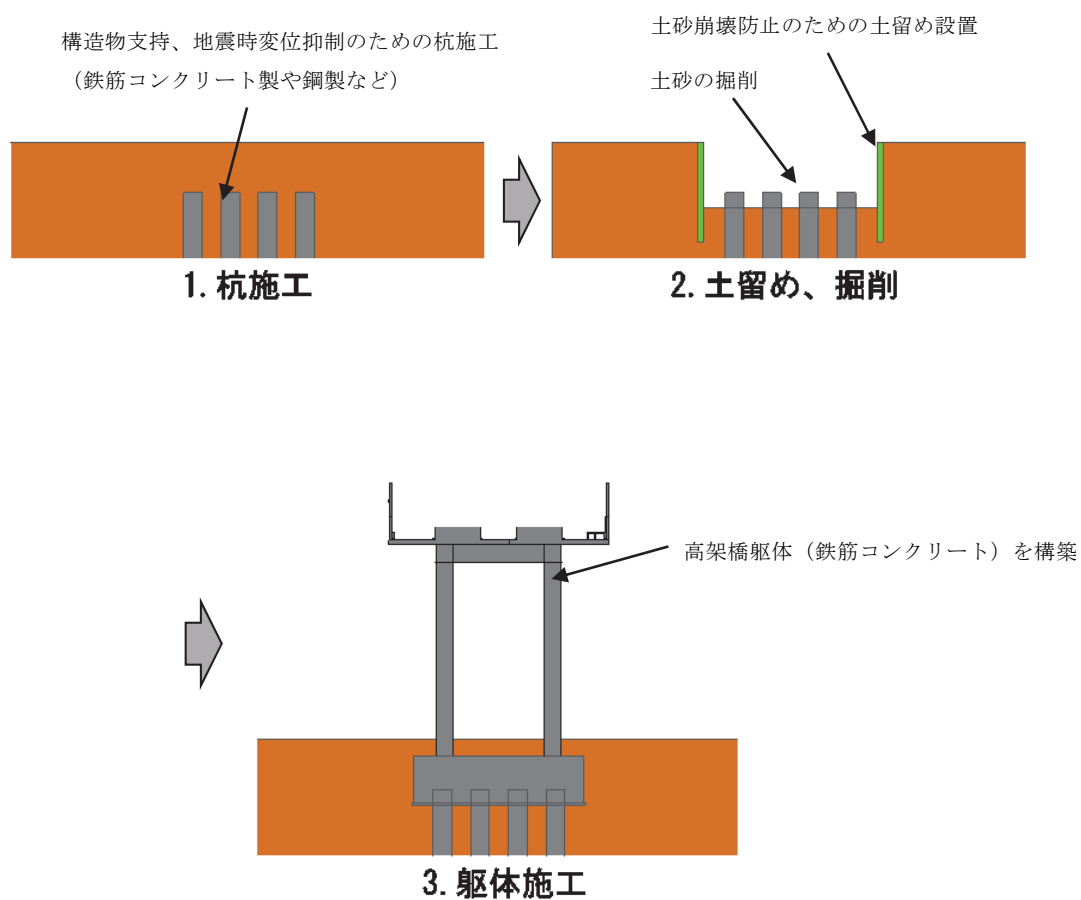
図 3-3-8 高架橋の施工イメージ ※場所打ち工法の場合
