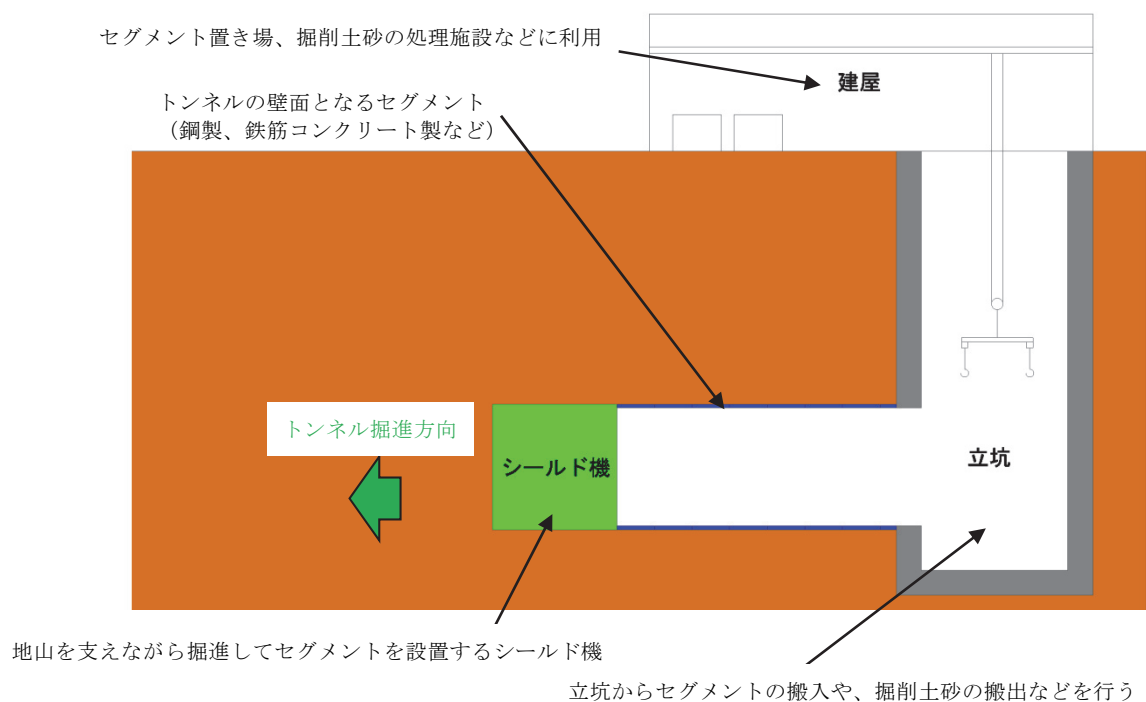
図 3-3-12 都市トンネルの施工イメージ ※シールド工法の場合
