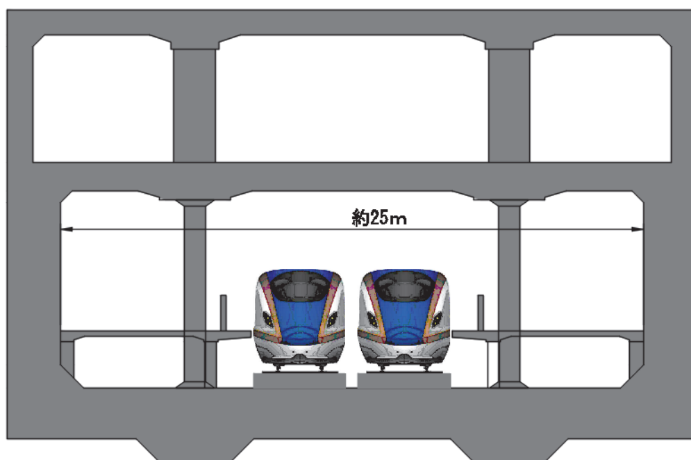
図 3-3-5 地下駅のイメージ ※2面2線の場合
