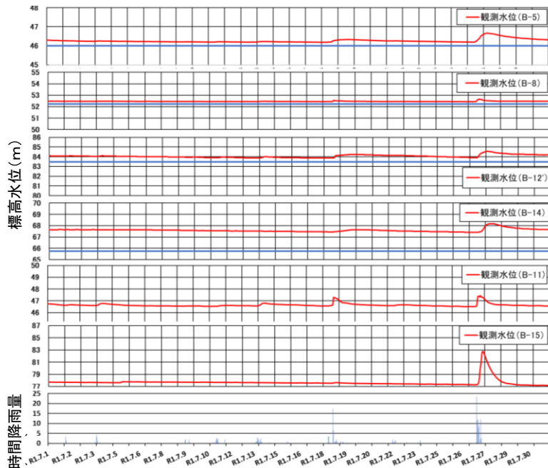
地下水位観測結果図(自記記録)
