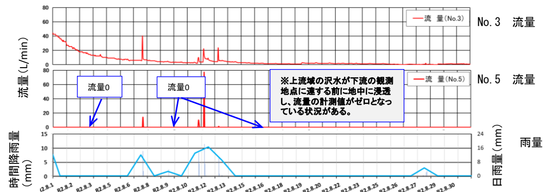
流量観測結果図(自記記録)
