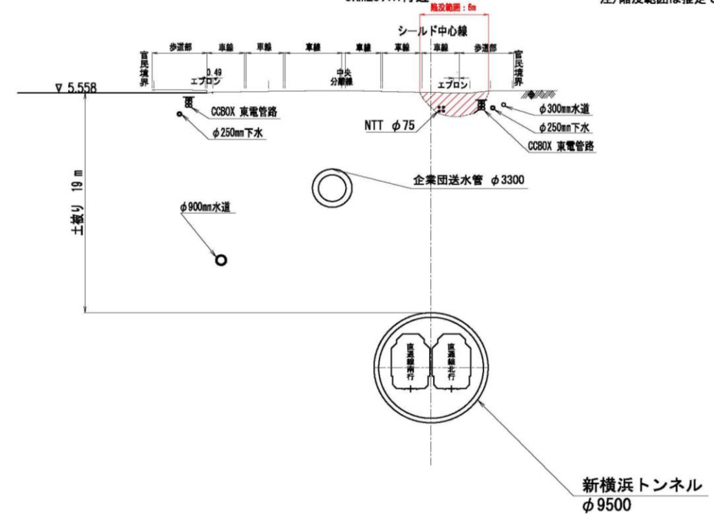
断面図
