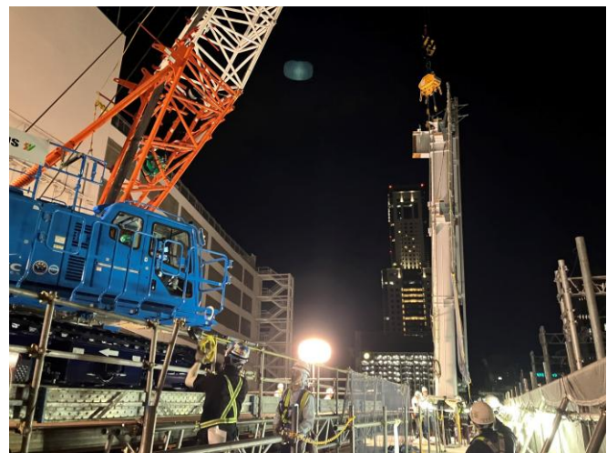
鉄骨建方工事の様子 最初に柱部材鉄骨の建て込みを90tクレーンを使用して行いました。
