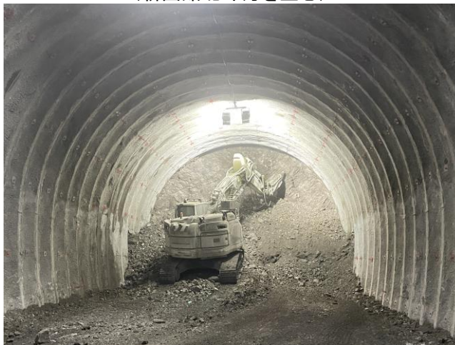
渡島トンネル(南鶴) トンネル掘削工施工状況 (新函館北斗方を望む)
