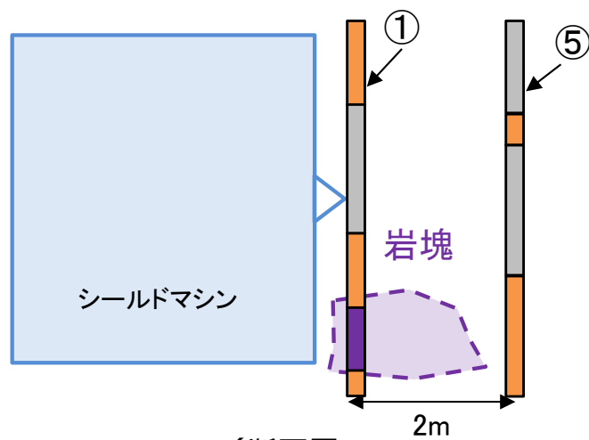
B-B' 断面図
