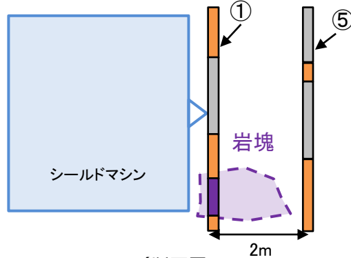
B-B'断面図
