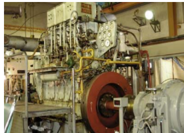
陸上エンジン試験機
