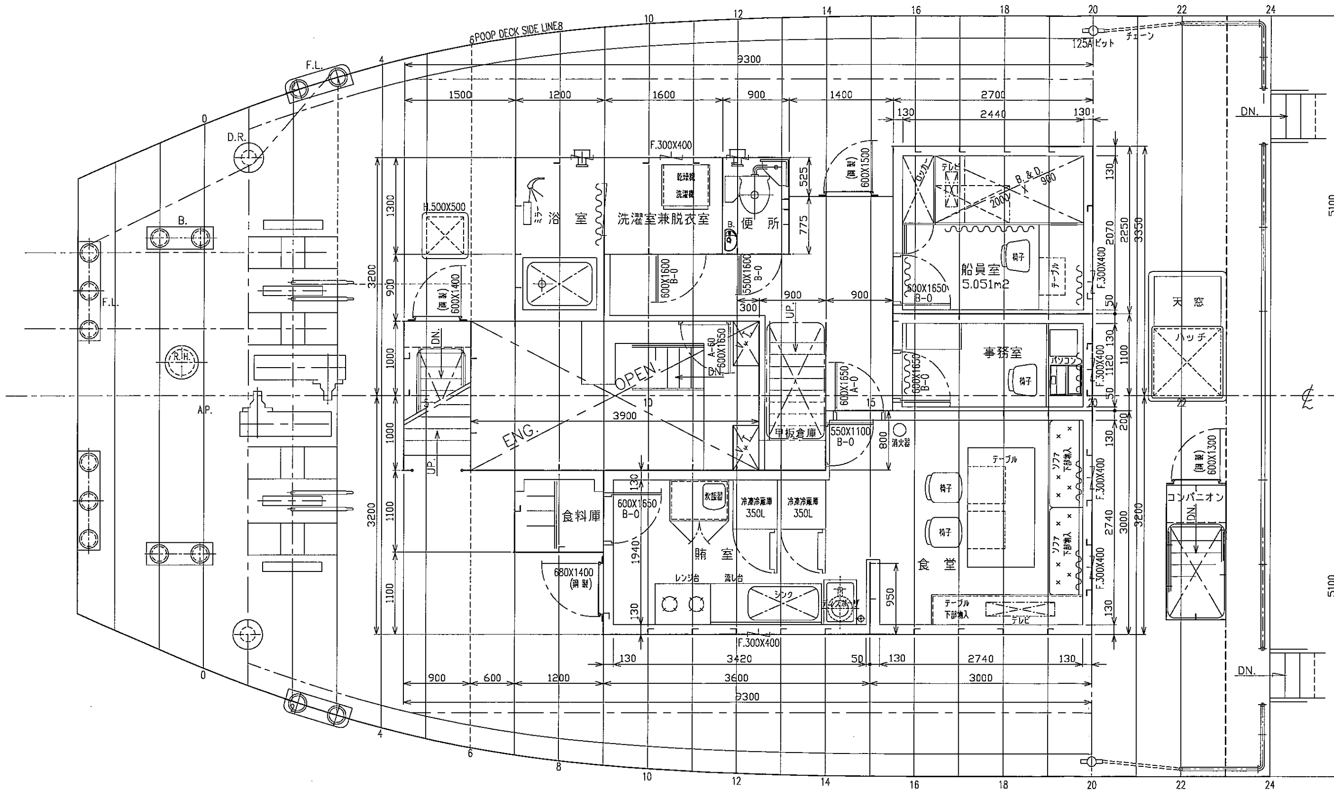
船尾楼甲板上配置図
