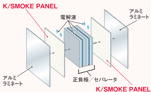
K/SMOKE PANEL 搭載リチウムイオン電池の構造
