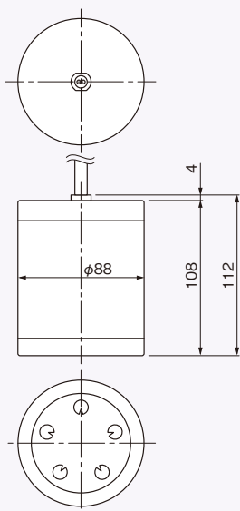
機器図面 (本体)
